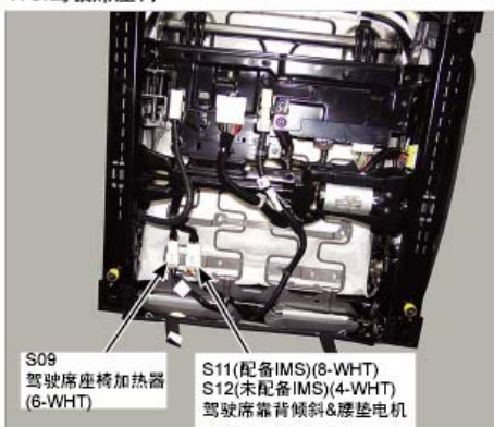
179. 驾驶席座椅
