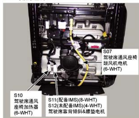
180. 驾驶席座椅
